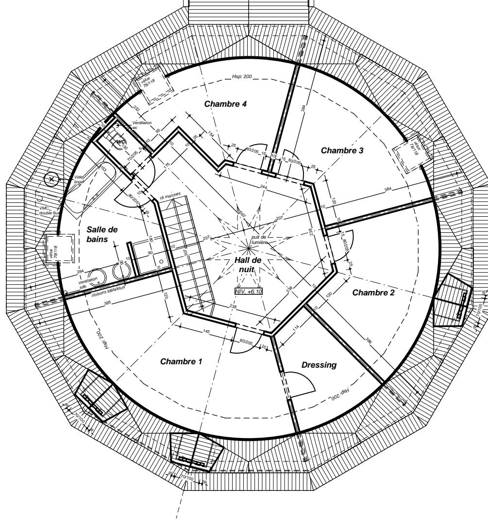
Etage 2 ( NIV. +6.10 )
